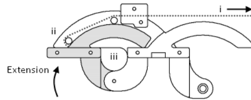
Fig. 14. Force feedback module
